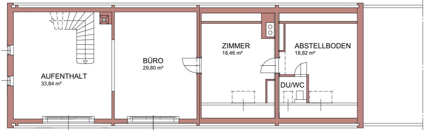
GRUNDRISS DACHGESCHOSS
