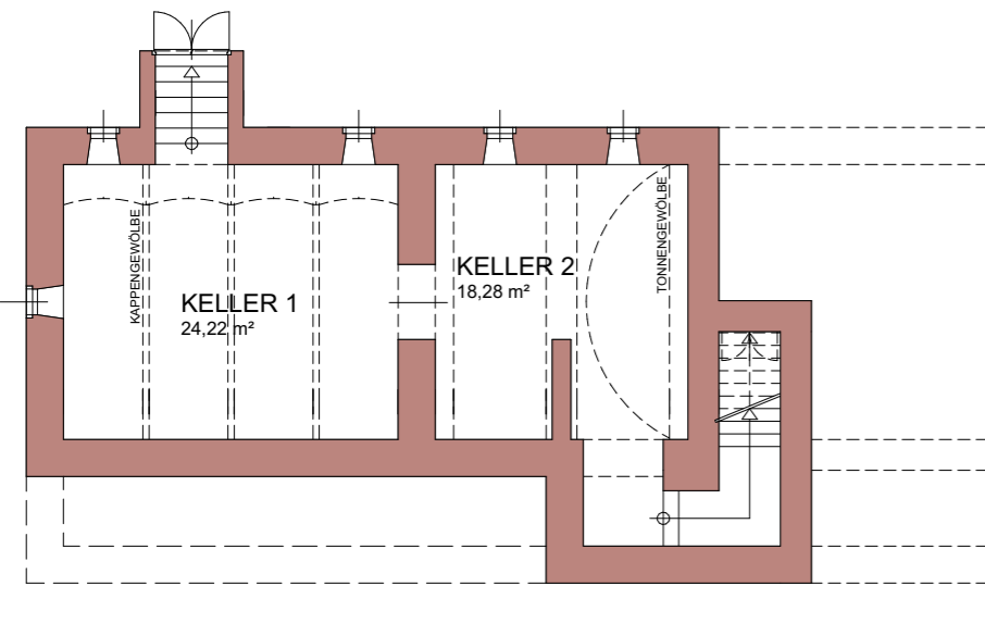
GRUNDRISS KELLER
